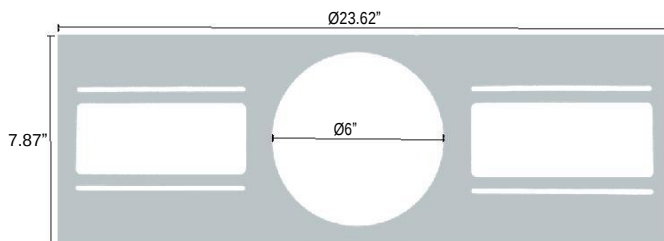
Plaque de montage 6po SL6-MP-R-V2
