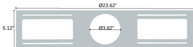
Plaque de montage 4po SL4-MP-R-V2
