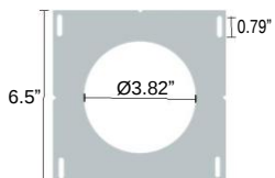
Plaque de montage 4po SL4-MP-R-V2
